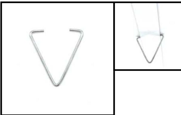
Dreieckshaken 37 mm lang, 1,5 mm ø verzinkt Art-Nr. 01-626037-01 Verpackungseinheit: 100 Stück 5,90 € per 100 Stück
