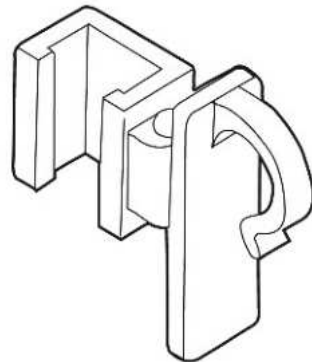
Aufhängehaken 2-teilig zum einhängen von Rahmen an Drahtgittern bis max. 12 mm Ø, grau Art-Nr. 08-100136-15 Verpackungseinheit: 10 Paar Preis: auf Anfrage
