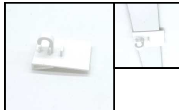
Deckenclip weiß 20 x 30 mm, mit Haken Art-Nr. 01-227700-05 Verpackungseinheit: 100 Stück 24,80 € per 100 Stück
