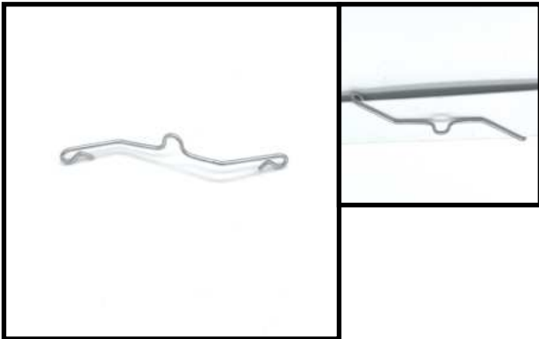
Deckenspinne 77 mm lang, 1,6 mm ø verzinkt Art-Nr. 01-570430-01 Verpackungseinheit: 100 Stück 7,90 € per 100 Stück
