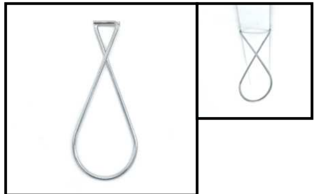
Deckenklemme 65 mm lang, 1,6 mm ø verzinkt Art-Nr. 01-618650-01 Verpackungseinheit: 100 Stück 8,00 € per 100 Stück
